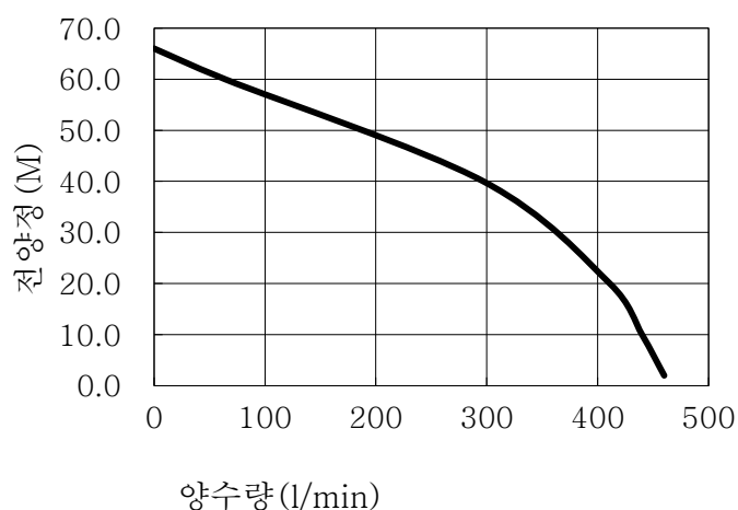
성능곡선도
